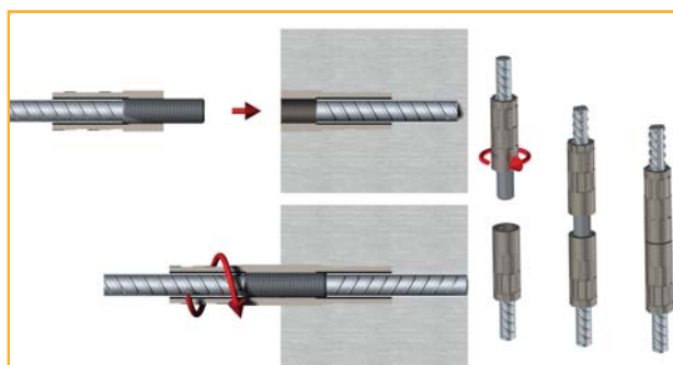
Figura 16: Montagem da emenda direita-direita
