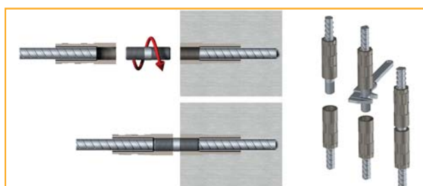
Figura 17: Montagem da emenda direita-esquerda
